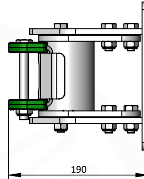
Montage / Mounting mini
